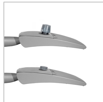
Dostępne z gniazdem NEMA lub Zhaga dla różnych opcji połączeń.
