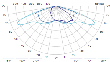
LENZO FLEX 4 50009
