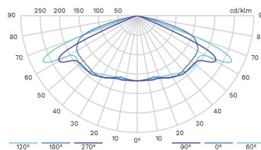
LENZO FLEX 4 50008
