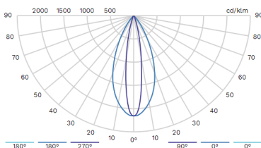
6933 Faisceau elliptique horizontal
