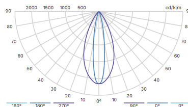
6934 Faisceau elliptique vertical
